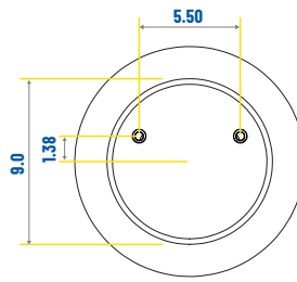
VISTA DE MONTAJE SUPERIOR
