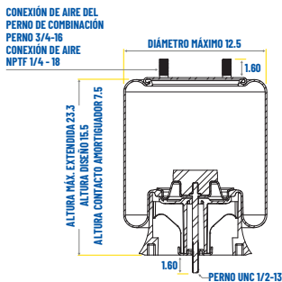
VISTA LATERAL DE ALTO Y ANCHO
