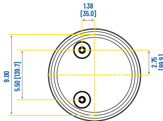
VISTA DE MONTAJE SUPERIOR
