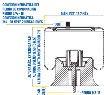
VISTA LATERAL DE ALTO Y ANCHO
