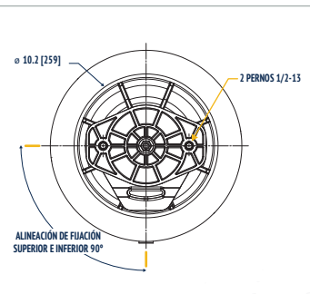
VISTA DE MONTAJE INFERIOR
