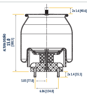
ALTURA Y ANCHO EN VISTA LATERAL
