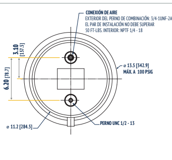
VISTA DE MONTAJE SUPERIOR
