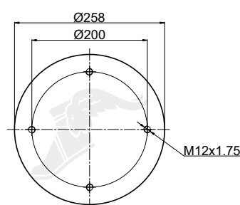
Piston
