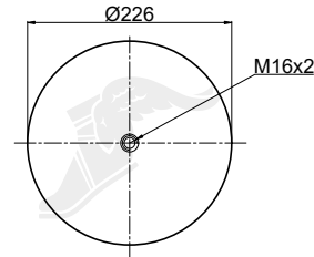
Piston
