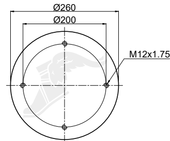
Piston
