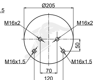
Piston
