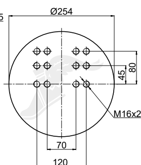
Piston
