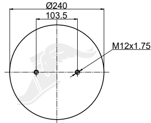
Piston
