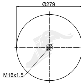
Piston
