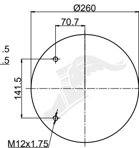
Piston
