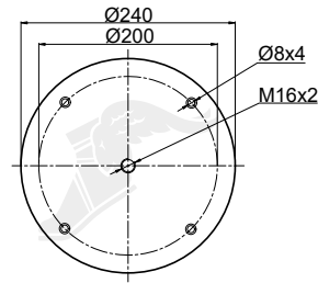
Piston
