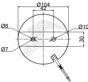
Piston
