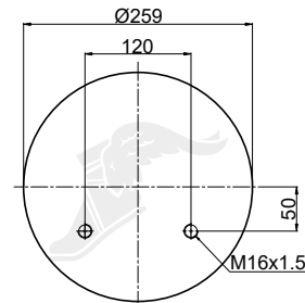
Piston
