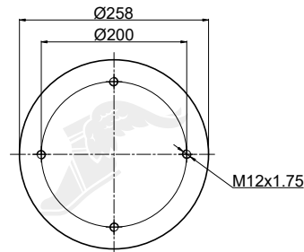
Piston
