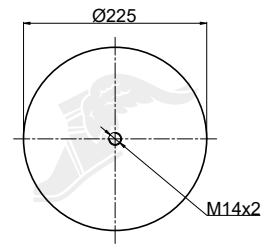
Piston
