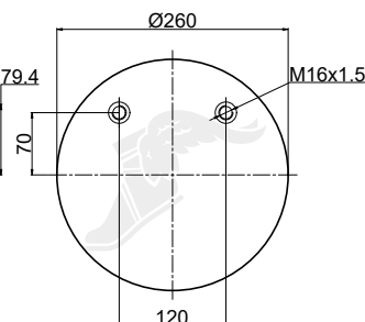
Piston
