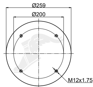
Piston
