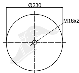
Piston
