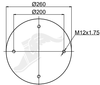
Piston
