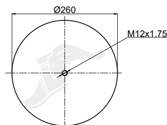
Piston
