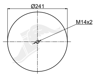
Piston
