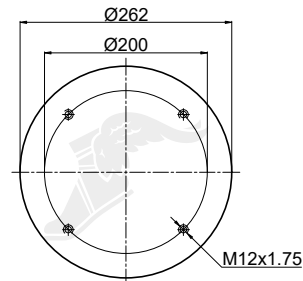
Piston
