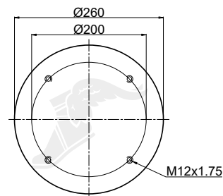
Piston
